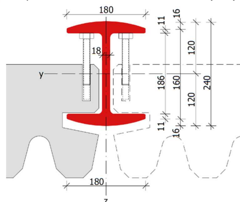
Coupe transversale et formats de base (mm)
